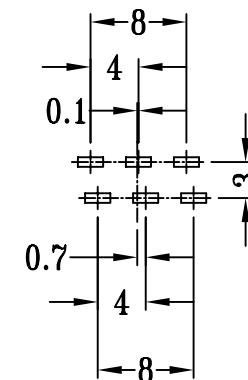
P.C.B LAYOUT
